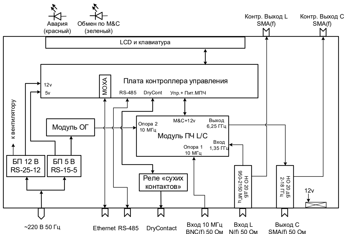
Рисунок 2 – Структурно-функциональная схема ПЧ «вверх»
